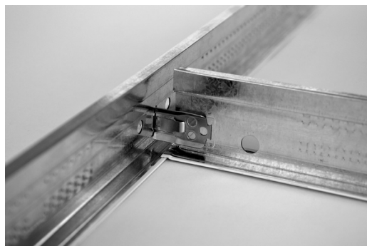
Deutliches Clickgeräusch beim einrasten
